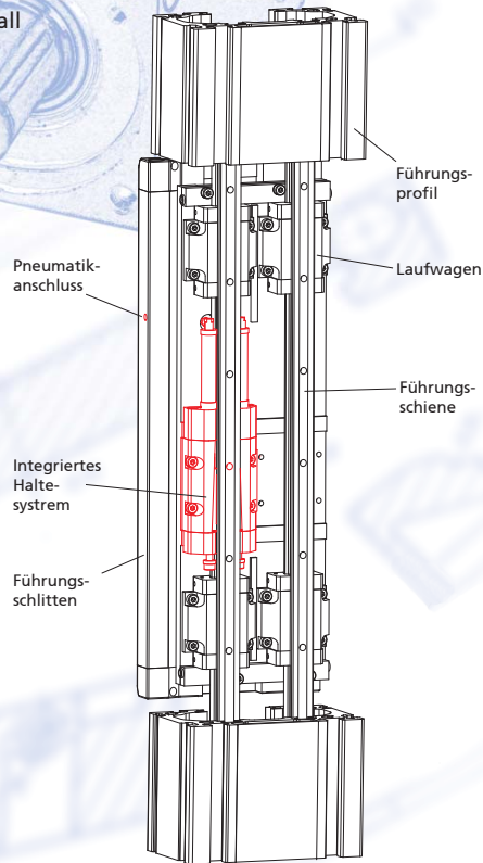
Grafik zeigt: Lastfall am Schlitten
